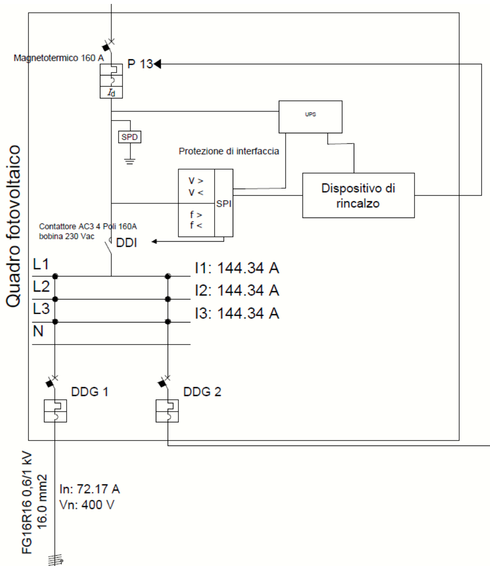
Fig. 19: Dettaglio SPI e DDI
