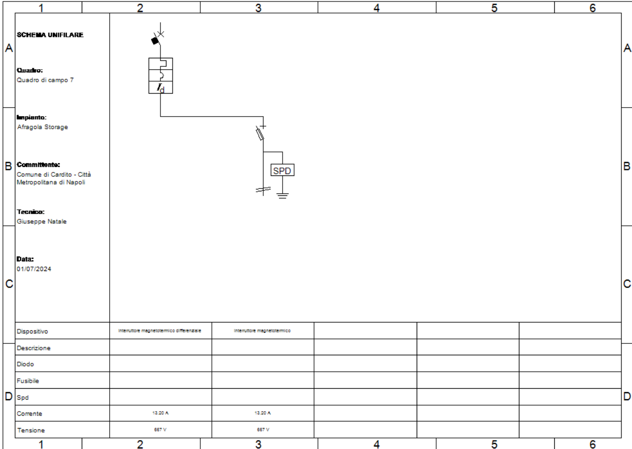
Fig. 12: Schema unifilare quadro "Quadro di campo 7"
