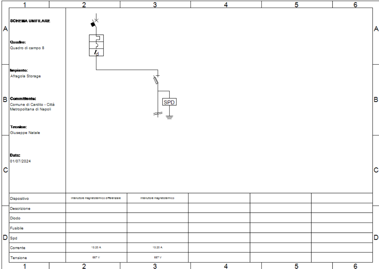
Fig. 13: Schema unifilare quadro "Quadro di campo 8"
