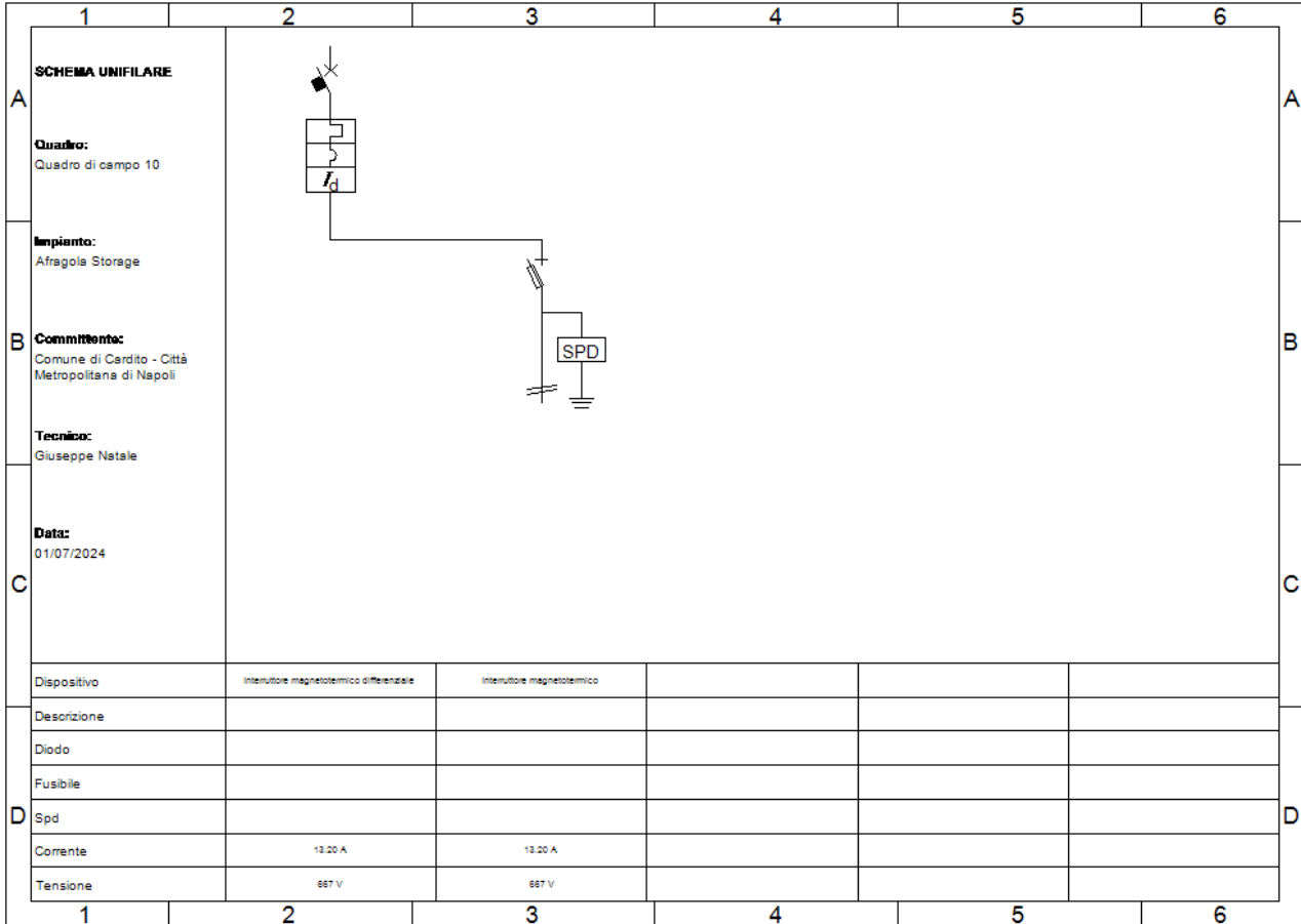
Fig. 15: Schema unifilare quadro "Quadro di campo 10"
