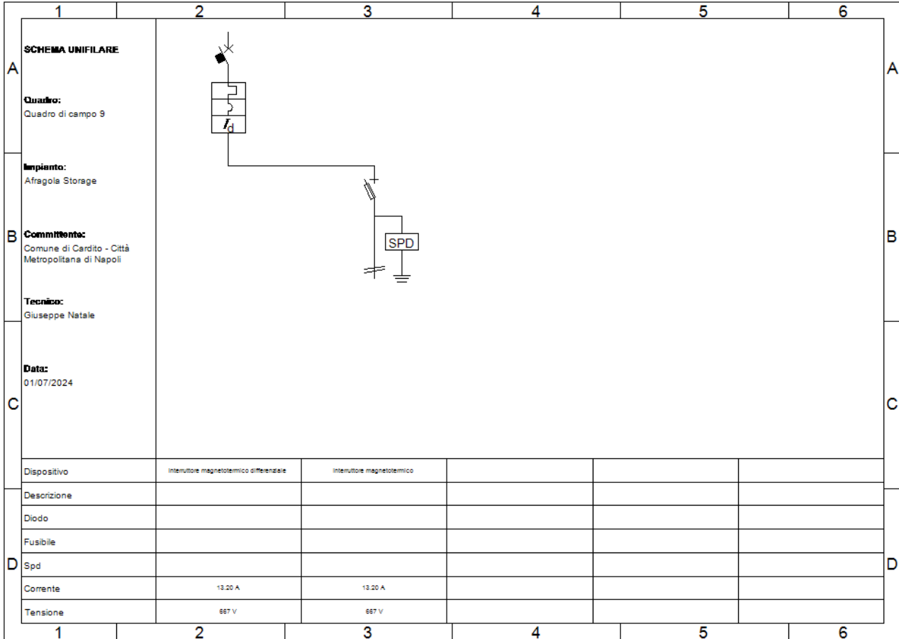
Fig. 14: Schema unifilare quadro "Quadro di campo 9"
